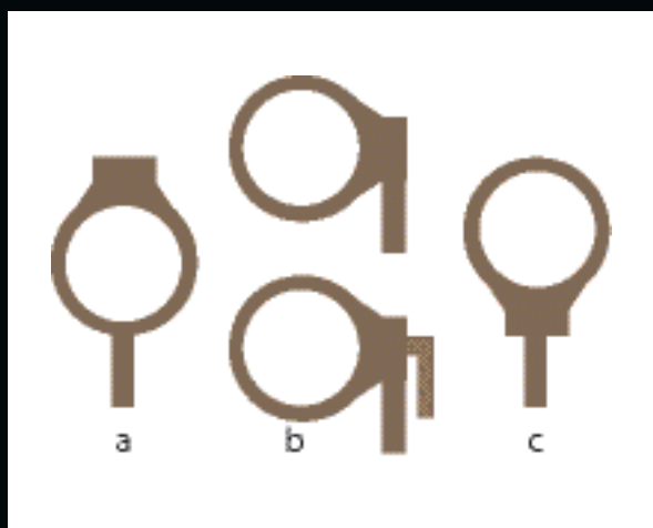
Рис. 7. Различные варианты присоединения литника к модели: неправильное (а) и правильное (б, в) соединения литников
