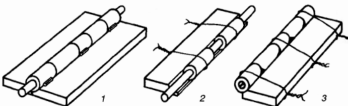
Рис. 2. Простой шарнир
