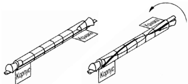
Рис. 3. Пружинящий шарнир.
